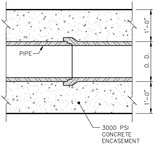
LONGITUDINAL SECTION
