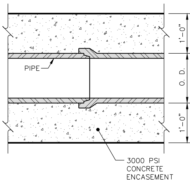
LONGITUDINAL SECTION
